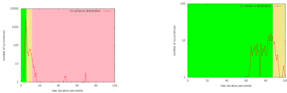
(b) Exemple d'un motif ne permettant pas de trouver des anomalies : q = 75\% incite à prendre tout l'intervalle [0..88\%] comme groupe de référence. s = 2 ne permet de trouver aucune anomalie
